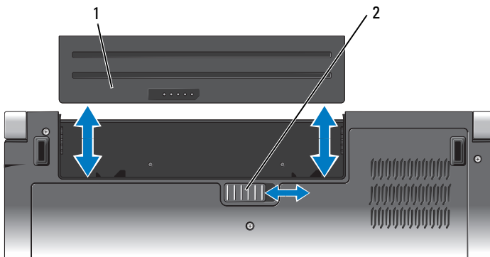
1 Akku 2 Akkufachfreigabevorrichtung
